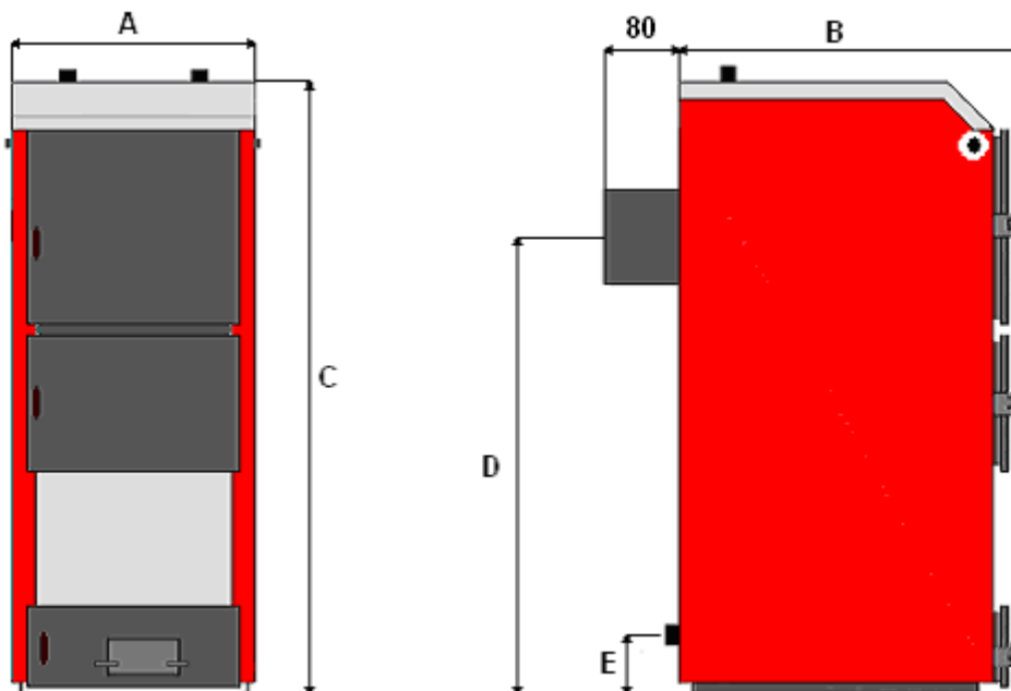
Rys. 2 Schemat poglądowy MINI
