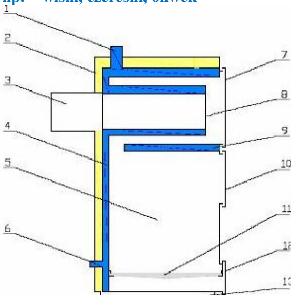
Rys. 1 Przekrój wzdłużny kotła MINI
