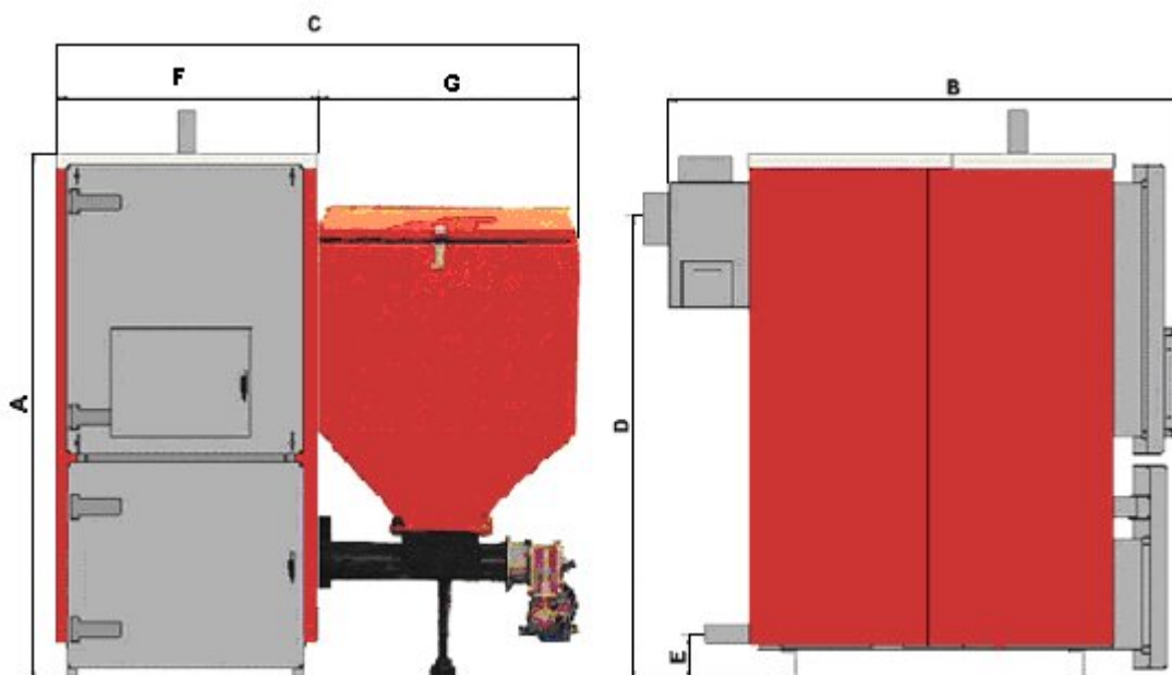
Rys. 2 Widok poglądowy kotła HEITZ MAX EKO
